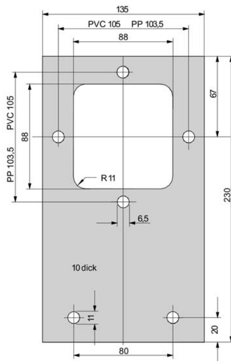
Halterungsplatte / mounting plate version
